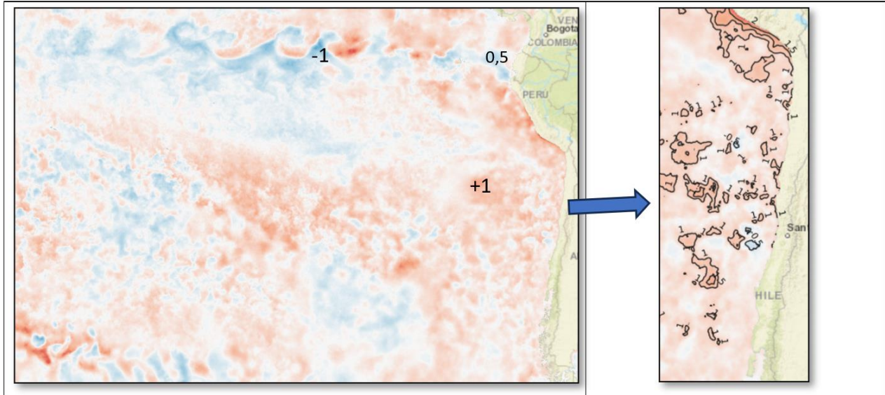
Figura 2. ATSM océano Pacífico- costa sudamericana del 25 de agosto de 2025. La información de ATSM fue extraída del producto MUR, calculadas en base a la climatología de TSM satelital del periodo 2002 – 2025, provenientes de la plataforma SAPO-Chile (IFOP).
